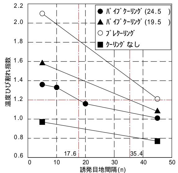
図 - 5 目地間隔と温度ひび割れ指数の関係
