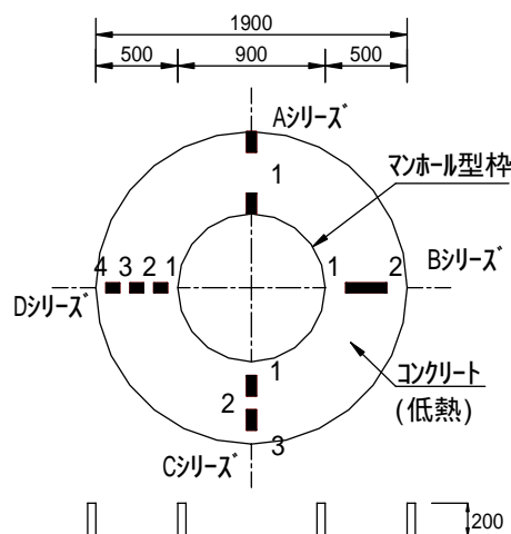
図 - 6 誘発目地の検討に使用する試験体
