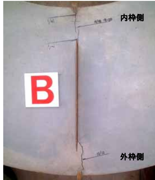
写真 - 1 62% B シリーズひび割れ発生状況
