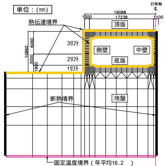
図 - 3 解析モデル図 (1/2 モデル)
