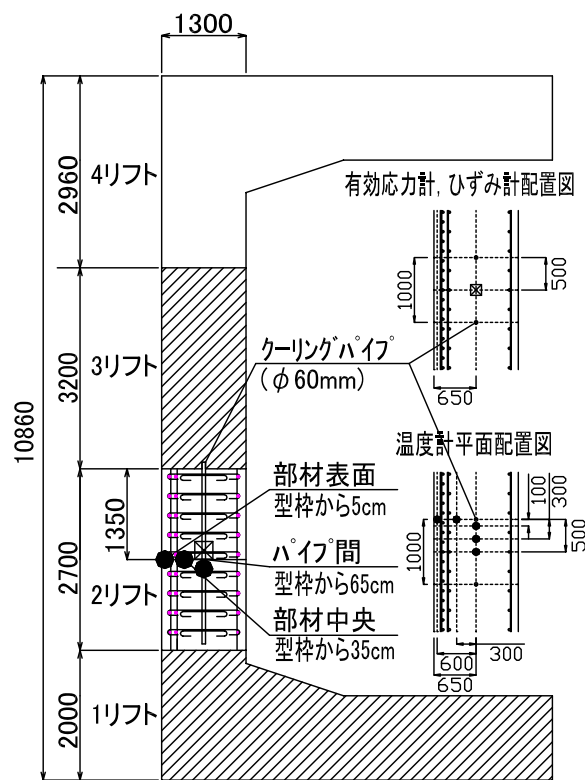
図-4 計測機器配置図 (B○x3北側壁)
